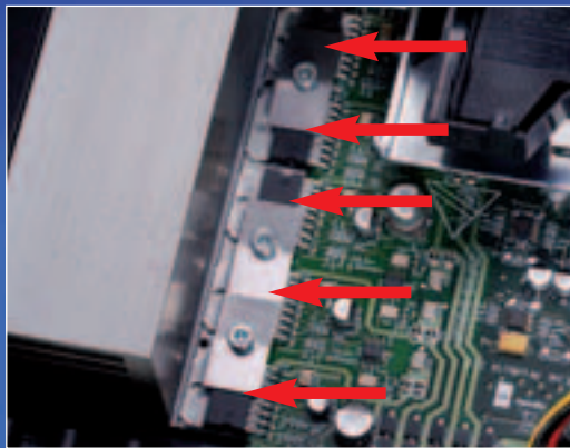
Bei den Endstufen verlassen sich die Linn-Ingenieure auf fünf ICs von ST Microelectronics (Pfeile).
