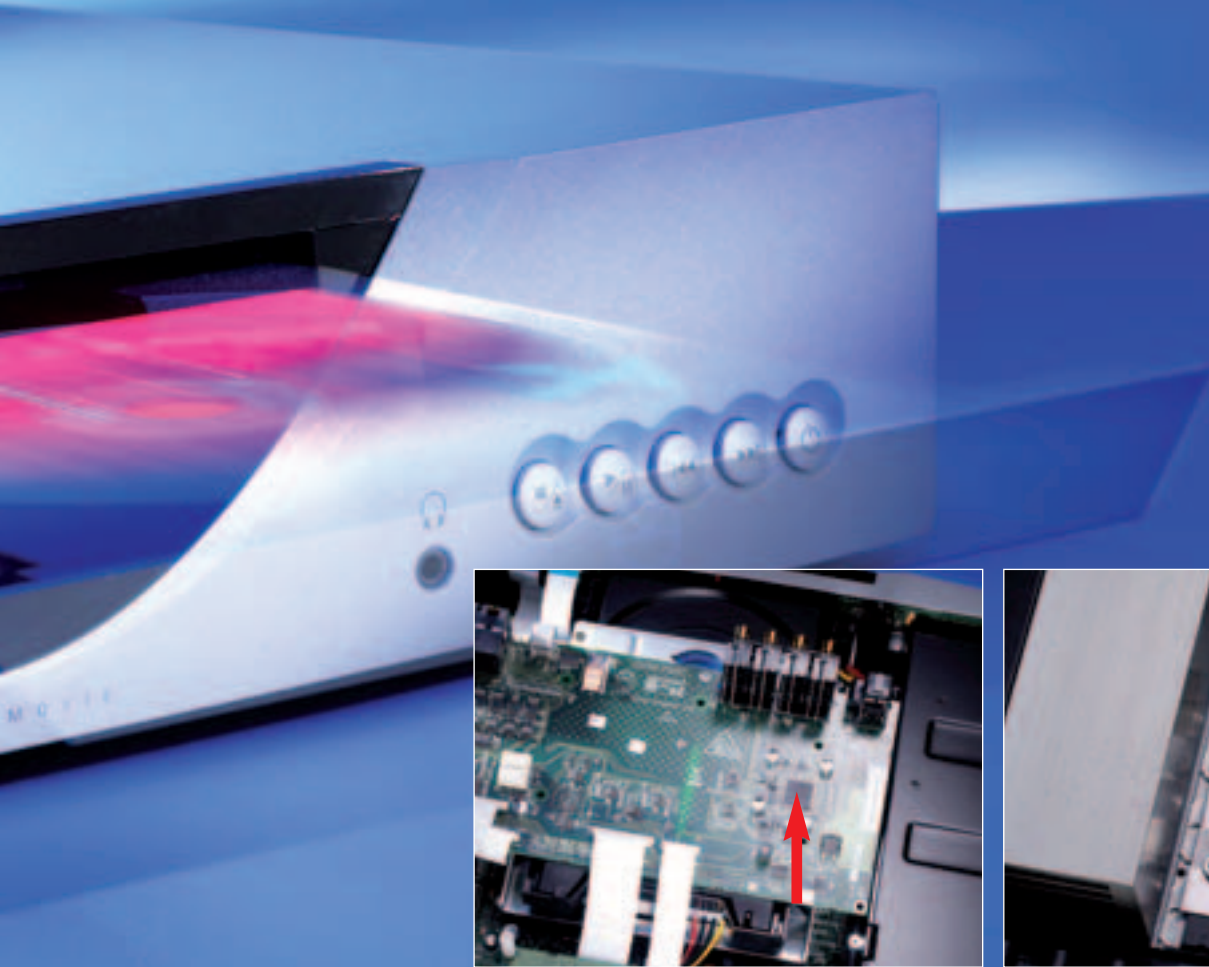
Die Videoabteilung bietet mit dem Matrix-IC von ST (Pfeil) keinen Normenwandler.
